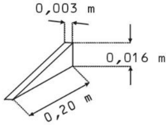
Detalle del refuerzo
