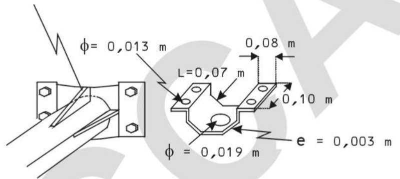
Detalle abrazadera
